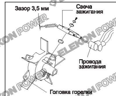
Рис. 17 Снятие свечи зажигания
