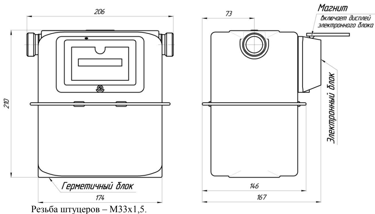
Рисунок 2 – Счетчик газа бытовой с электронным термокомпенсатором СГБЭТ G4-1 или СГБЭТ G2,5-1
